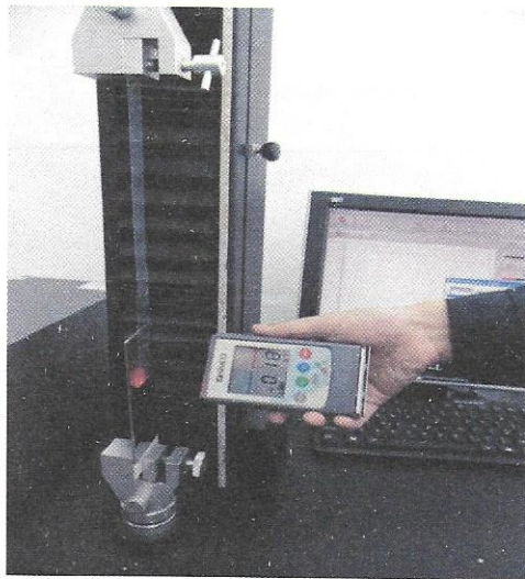
图2 胶粘带剥离电压测试示意图
